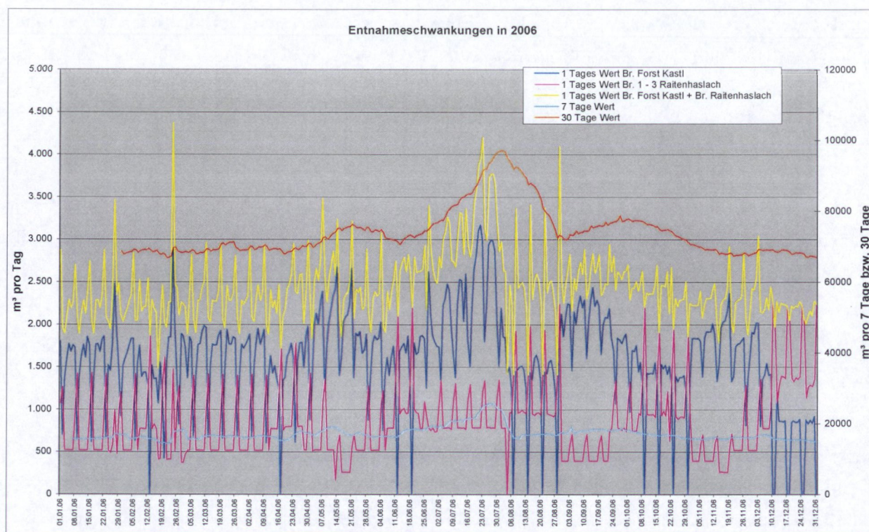
Abb. 1: Tägliche Fördermengen aus den Brunnen der Gde. Burgkirchen in 2006
